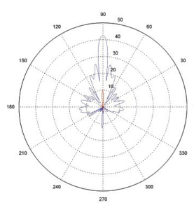
5.5 Ghz H-Plane and E of H-plane
